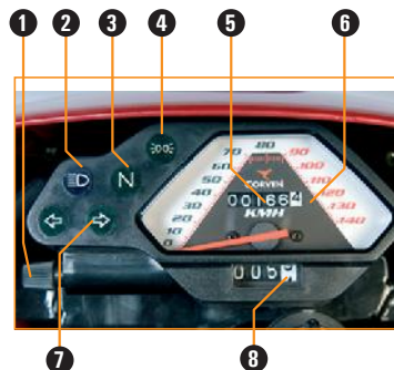
Fig.5 Instrumentos e indicadores
