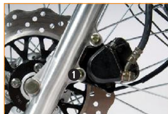
Fig.26 Caliper y disco de freno
